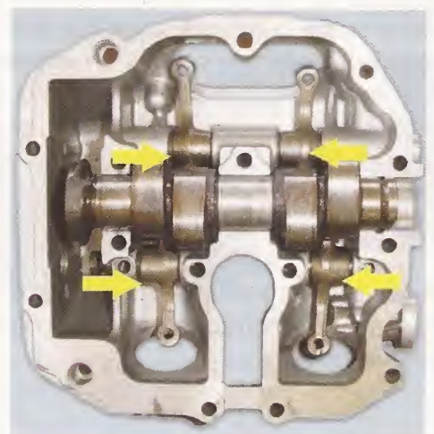
Balancines en contacto
